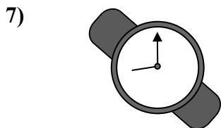
Наручные часы
